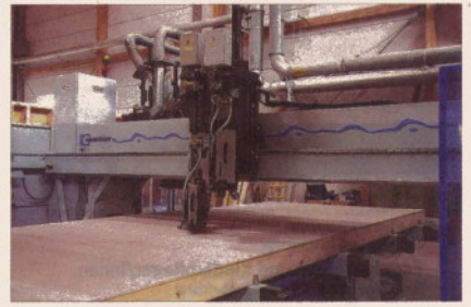
Die neue Fertigungslinie kann jetzt auch Säge-, Bohr- und Fräsarbeiten übernehmen. Fotos: Jan Zawadil
